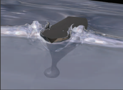
船模顶浪运动流场
