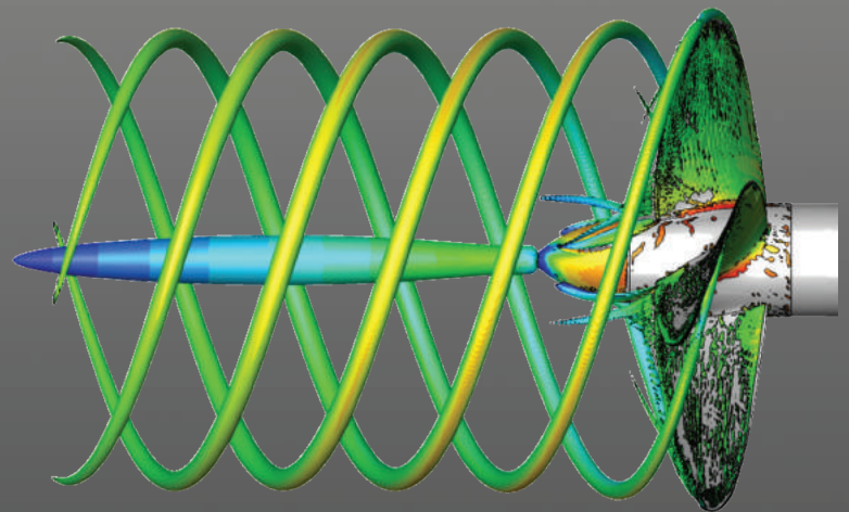
螺旋桨梢涡捕捉
