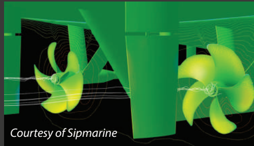
自航快艇尾迹
